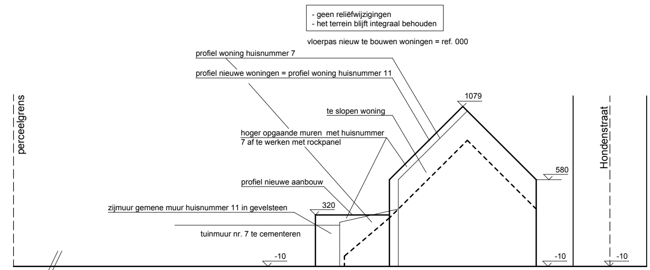
PROFIELSNEDE 1/250
