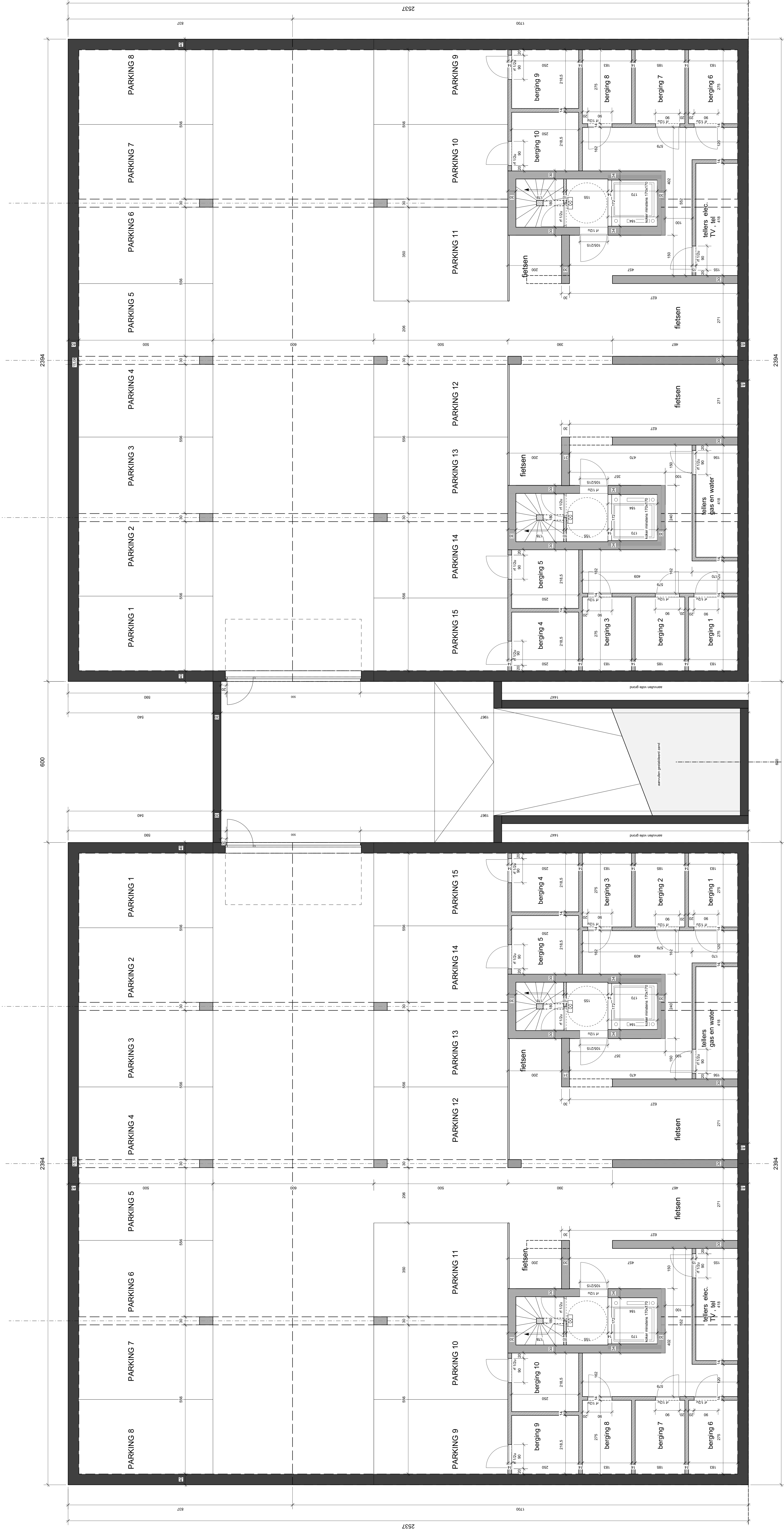
AZALEA STRAAT: KELDER 1/50
